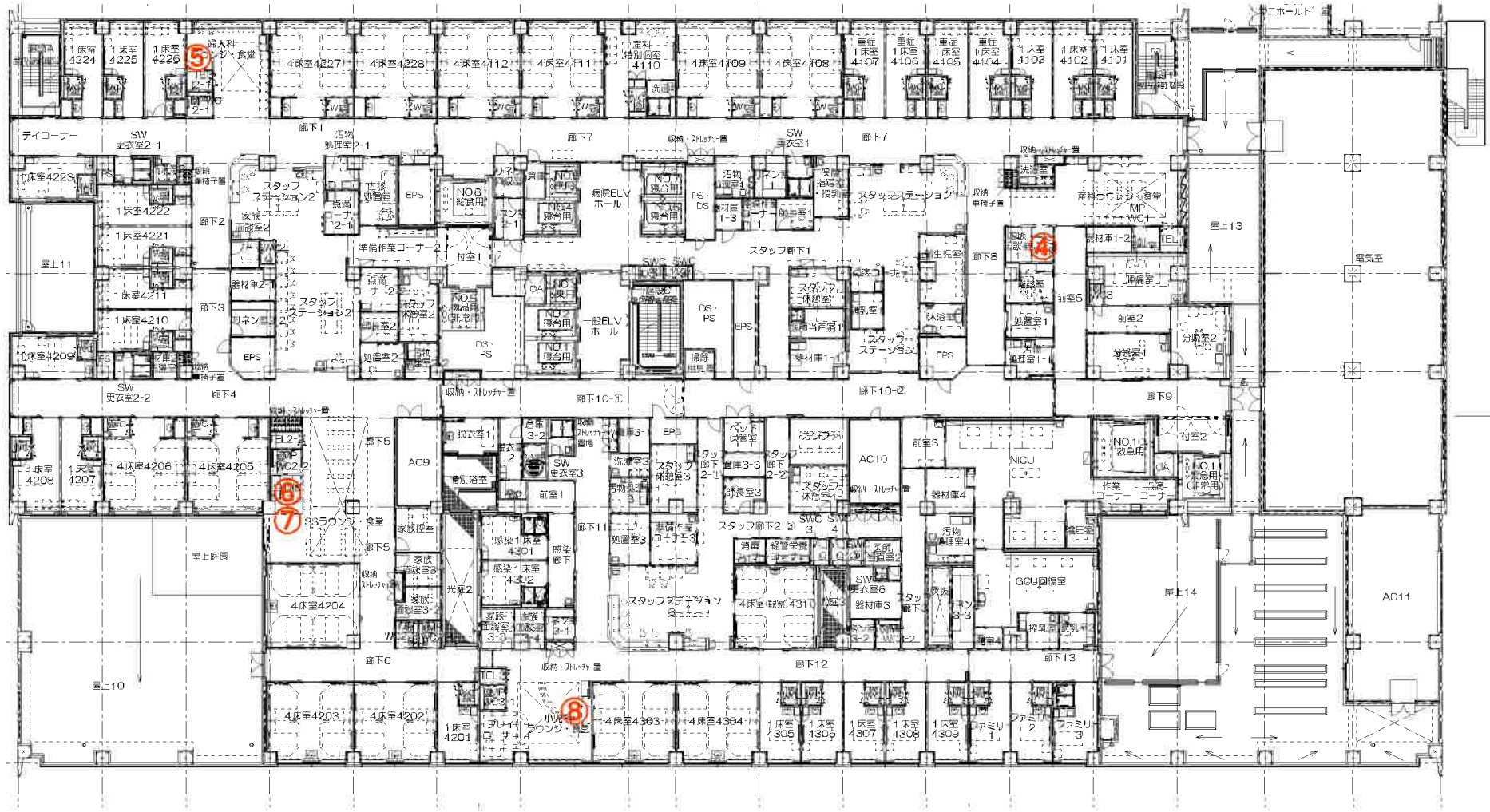
4階平面図
